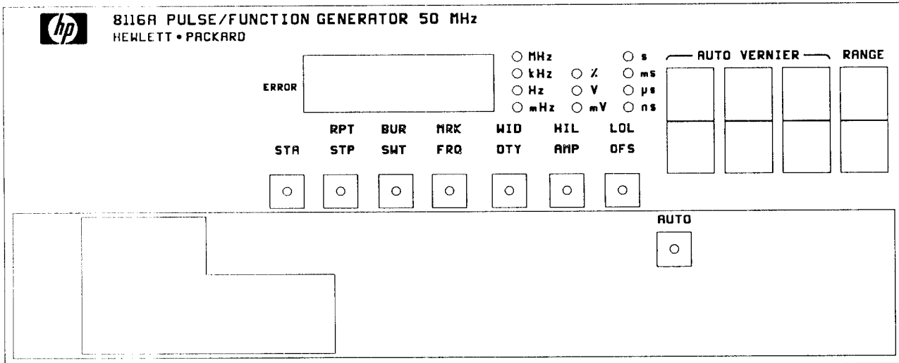
Figure 4-10. Parameter controls
